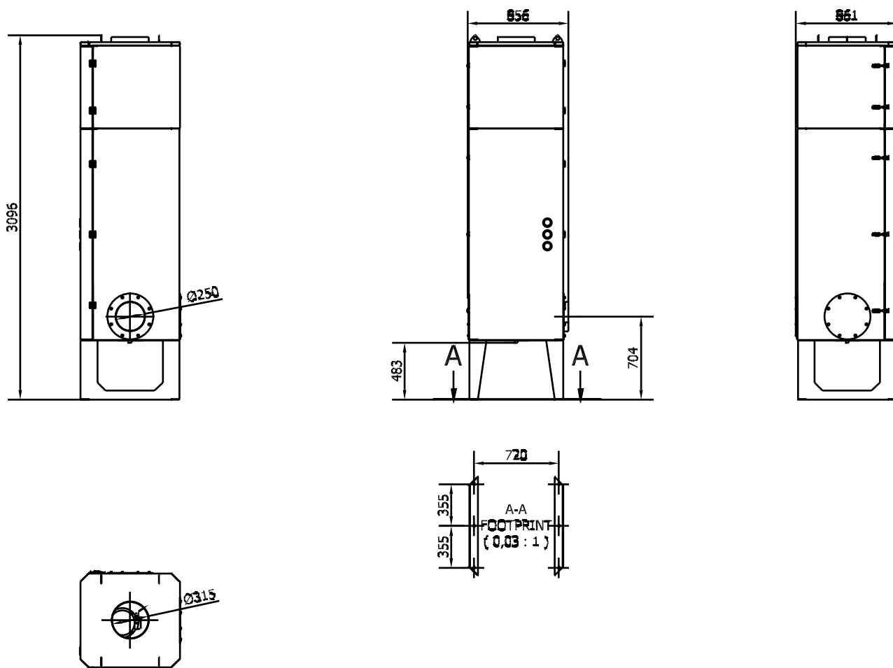
Ölnebelabscheider Typ OUPC 2020:
