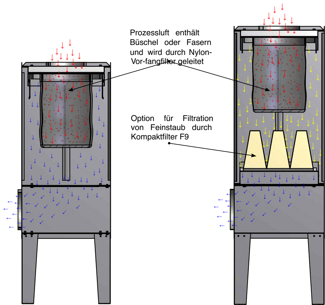
Prinzipskizze für Flow durch Vorfilterereinheit Typ SPC mit Vorfangfilter:
