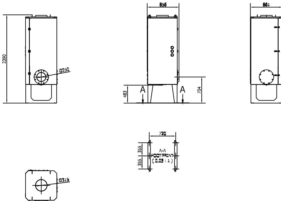
Ölnebelabscheider Typ OUPC 2020:
