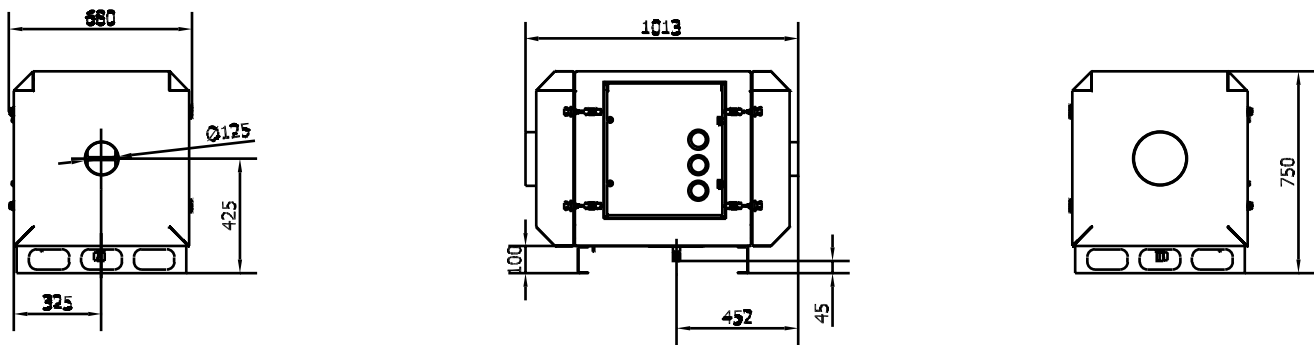
Ölnebelabscheider Typ OUPC 510:
