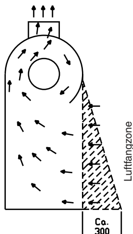
Modell B Turbowand mit gekrümmter Rückwand, um die Saugleistung zu optimieren.
