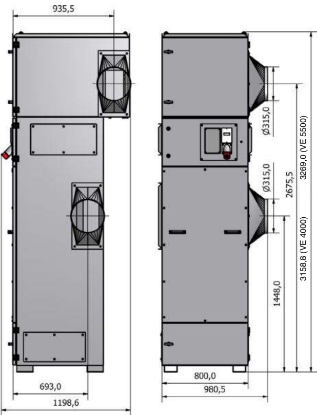
Filterline Typ FL 52H/VE 4000+5500:
