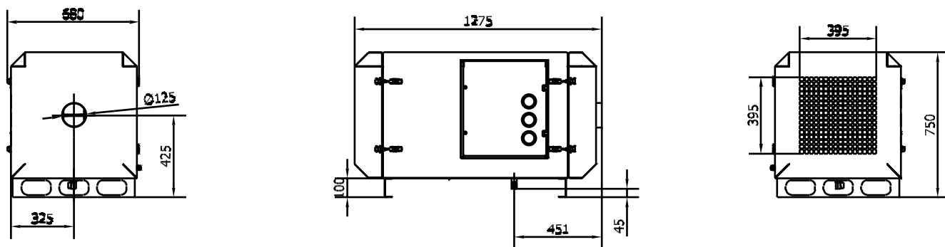
Ölnebelabscheider Typ OUPC 1000:
