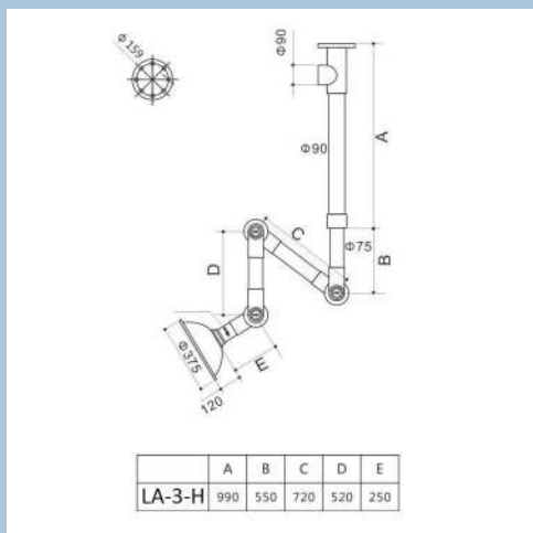
Absaughaube mit Gelenk.
